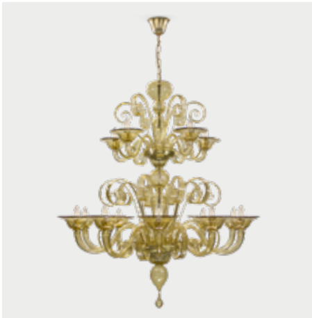
D0550-10+5-F Ø 110 cm - H 120 cm - C 55 cm - R 14 cm E14 15 x MAX 60W 18 KG
